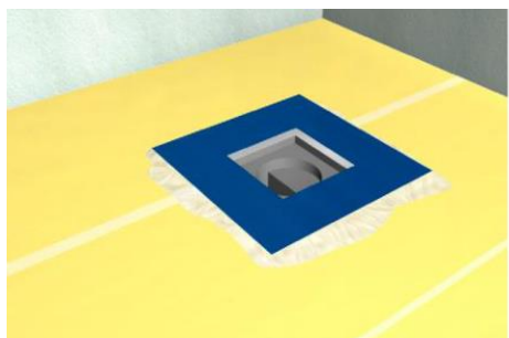
3 Шаг После завершения подготовки поверхности душевой лоток укладывается на пол с фильтром, бутиловая лента приклеивается к полу и прижимным роликом обеспечивается ее приклеивание к полу.
