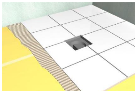
4 Шаг Нанесение керамики можно начинать после завершения нанесения изоляции.
