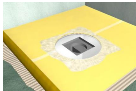
2 Шаг Подготавливают душевой канал, разрезая бутиловую ленту подходящего размера вокруг фильтра или сливного устройства.
